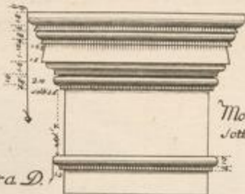
Capitello delli Pilastri lettera A.
