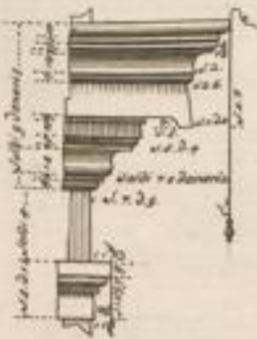
Bave del primo Imbasamento Lettera F.
