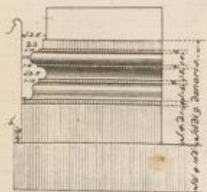
Dimostrazione delli Modini del passato foglio N.º 3 di dentro la Libreria Laurenziana.
