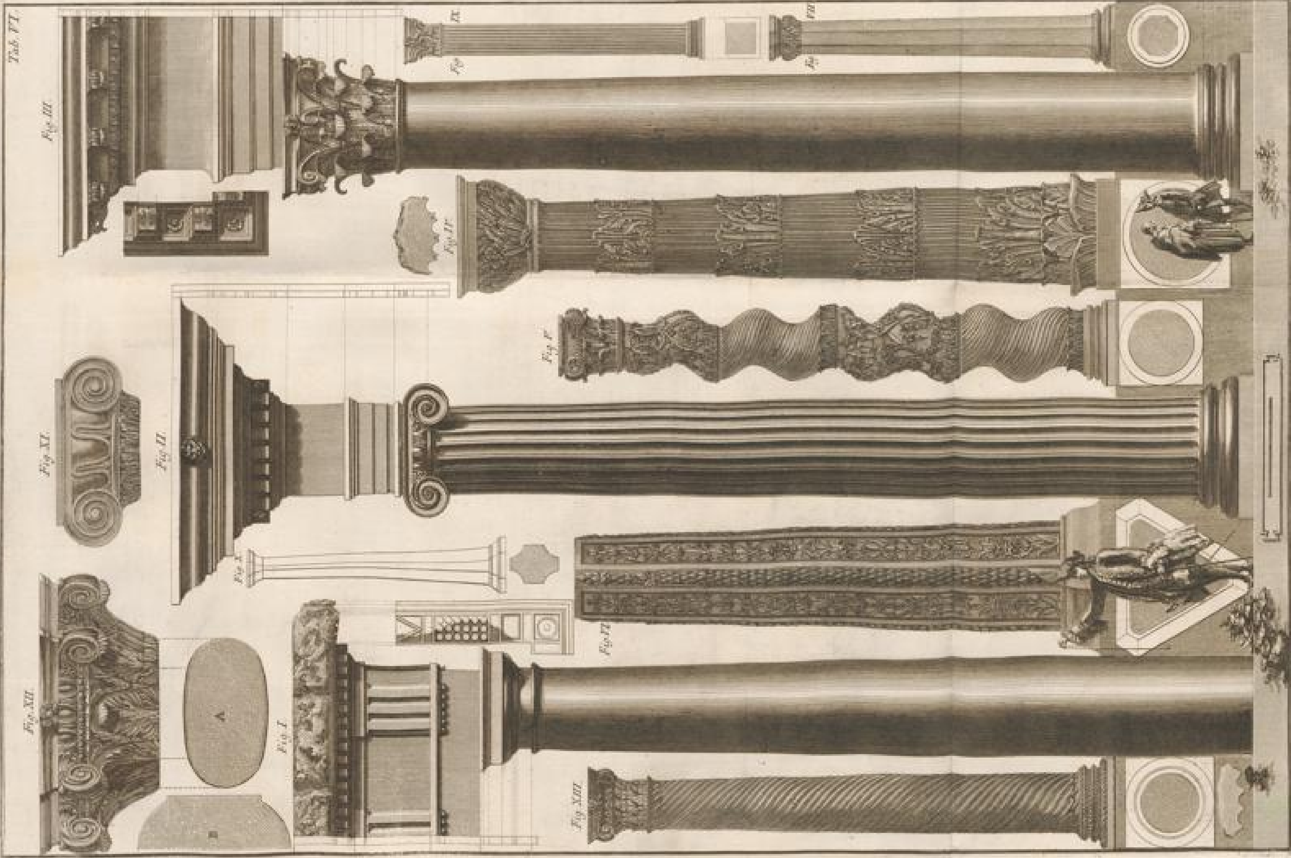
Partes in Architectura graecanica rationes ac symmetricae ex antiquis monumentis excerptae Fig. I. Columna doricae theatri Marcelli. Fig. II. Columna doricae aedae Fortunae Urbis nuncupatae. Fig. III. Columna corinthia in promae Partheni. Fig. IV. Columna corinthia in aedae Therae Praetoriae. Fig. V. Columna in cella SS. Crucis in Basilica Vaticana. Fig. VI. Columna triangularis in villa Beltonia ad Forum Subarvium. Fig. VII. Columna octogona in claustra Lateranensis aedae. Fig. VIII. Columna octogona in claustra Lateranensis aedae. Fig. IX. Columna octogona in claustra Lateranensis aedae. Fig. X. Columna octogona in claustra Lateranensis aedae. Fig. XI. Columna octogona in claustra Lateranensis aedae. Fig. XII. Columna octogona in claustra Lateranensis aedae. Fig. XIII. Columna octogona in claustra Lateranensis aedae. Fig. XIV. Columna octogona in claustra Lateranensis aedae. Fig. XV. Columna octogona in claustra Lateranensis aedae. Fig. XVI. Columna octogona in claustra Lateranensis aedae. Fig. XVII. Columna octogona in claustra Lateranensis aedae. Fig. XVIII. Columna octogona in claustra Lateranensis aedae. Fig. XIX. Columna octogona in claustra Lateranensis aedae. Fig. XX. Columna octogona in claustra Lateranensis aedae. Fig. XXI. Columna octogona in claustra Lateranensis aedae. Fig. XXII. Columna octogona in claustra Lateranensis aedae. Fig. XXIII. Columna octogona in claustra Lateranensis aedae. Fig. XXIV. Columna octogona in claustra Lateranensis aedae. Fig. XXV. Columna octogona in claustra Lateranensis aedae. Fig. XXVI. Columna octogona in claustra Lateranensis aedae. Fig. XXVII. Columna octogona in claustra Lateranensis aedae. Fig. XXVIII. Columna octogona in claustra Lateranensis aedae. Fig. XXIX. Columna octogona in claustra Lateranensis aedae. Fig. XXX. Columna octogona in claustra Lateranensis aedae.
